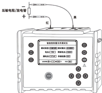
1.压敏电阻测试连接示意图
