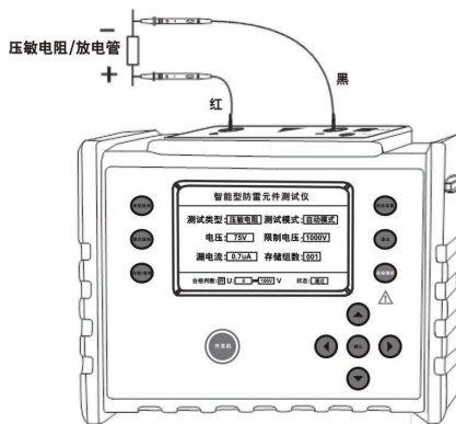
2.放电管测试连接示意图
