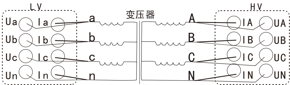
图 7.2.6 低压助磁三相测试接线图
