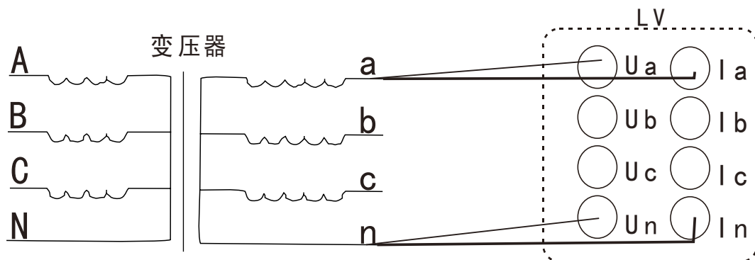
图 7.2.3 单相测试接线图
