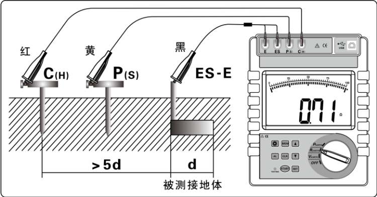
图 6（三线测试接地电阻示意图）
