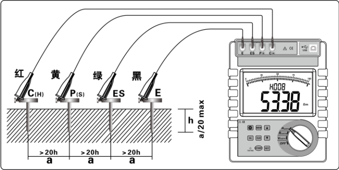
图 8（土壤电阻率测试示意图）
