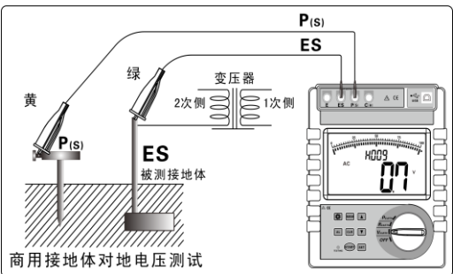
图 10（接地电压测试示意图）
