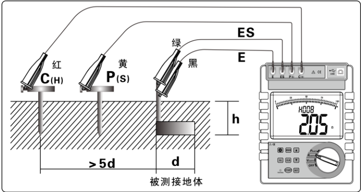
图 3 (四线精密测试接地电阻示意图)
