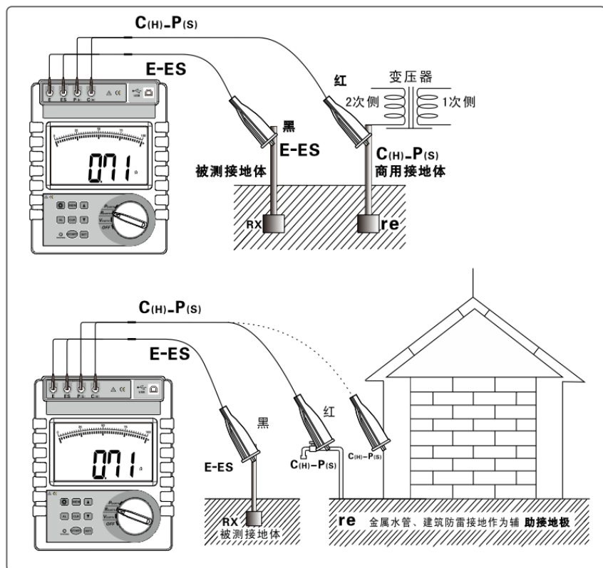
图 7（二线简易测试接地电阻示意图）
