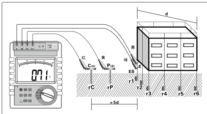
图 4（四线精密测试接地电阻示意图）
