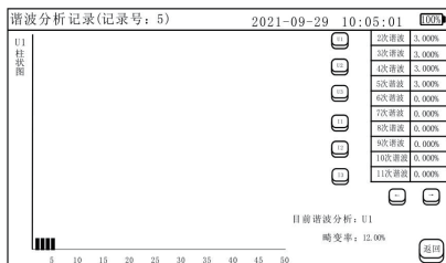
图 15 (谐波分析记录界面)
