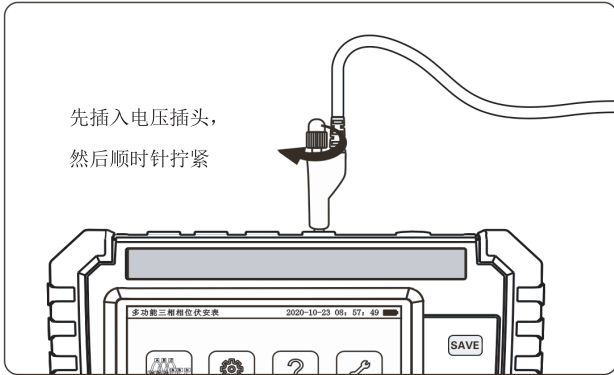
图 1 （电压测试线接法）
