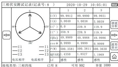
图 14 (三相伏安测试记录界面)
