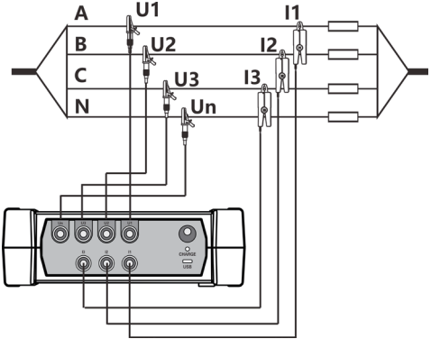
图 2 (Y 型接线)
