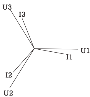
三相四线向量图
