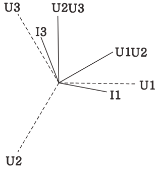
三相三线向量图
